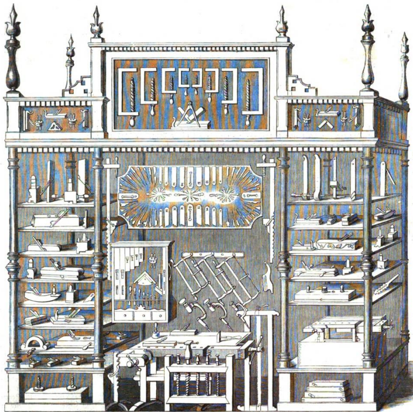
312. Werkzeuge von Joh. Weiß und Sohn in Wien.
