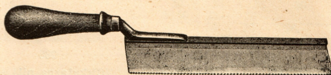
227 Listarica sa hrptom savinuta za furnire sa sitnim zubima
