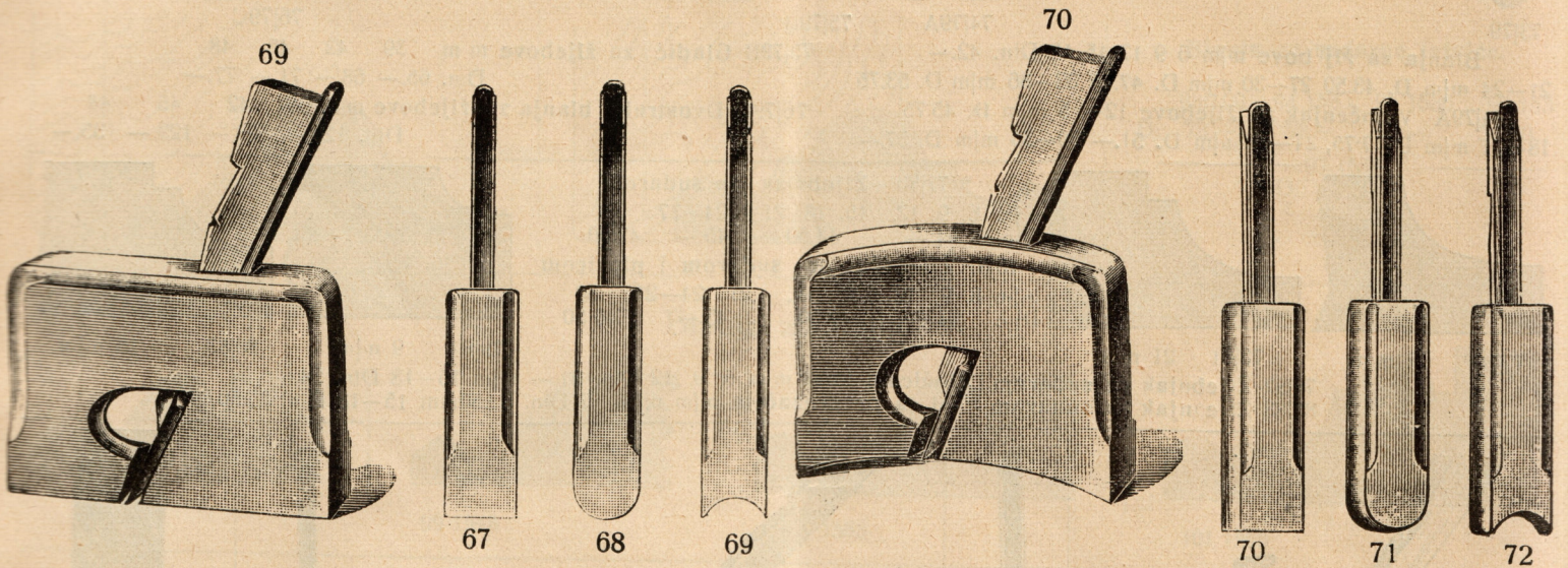
Ravni žljebnjaci oblika širina m/m Vjenac žljeb motka 6 9 12 15 18 21 komad D 38 —
