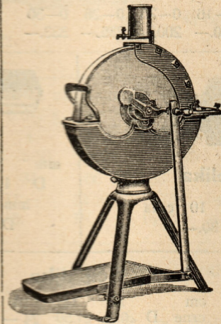
Brusevi, okrugli montirani u željeznom stalku sa zaštitnim limom i karticom 50 cm. prom- jera. Osobito priklan na za sve radionice stolara, tesara, toka- ra i kolara. D 1850.—
