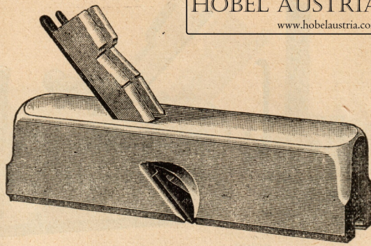
38|33 Bianja za prozore sa dva žej-za za poprili deb- ljina drva 30 mm (1-1 1/4) u obliku A, B, C, D. D 92.—
