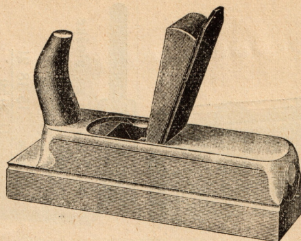
10|9 1/2. Zubna blanja sa okomitim željezom
