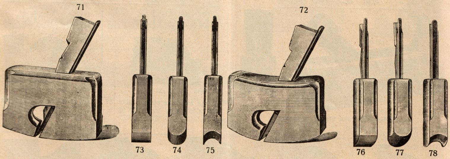
Zavinuti žljebnjaci oblika Vjenac žljeb motka širina m/m 6 9 12 15 18 21 komad D 47 —
