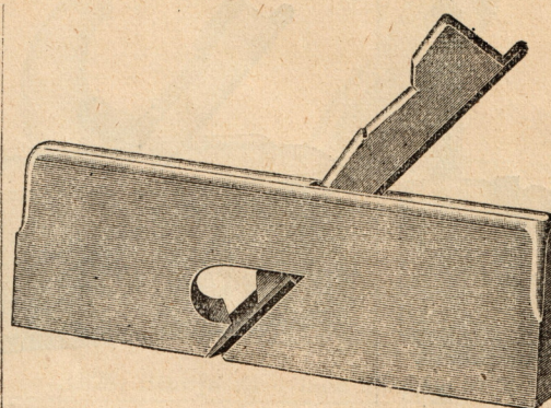
12|11 Vjenčanjak sa kosim željezom mm 9 12 15 18 21 D 38·25 mm 24 27 30 33 36 D 40·50 41·50 43— 46— 46—
