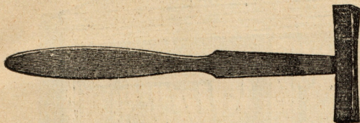
355 Staklarski čekić iz I-a čelika kovani sa drškom D. 17.—
