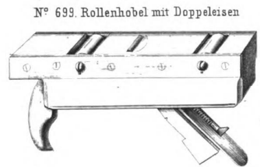
N° 699. Rollenhobel mit Doppelleisen
